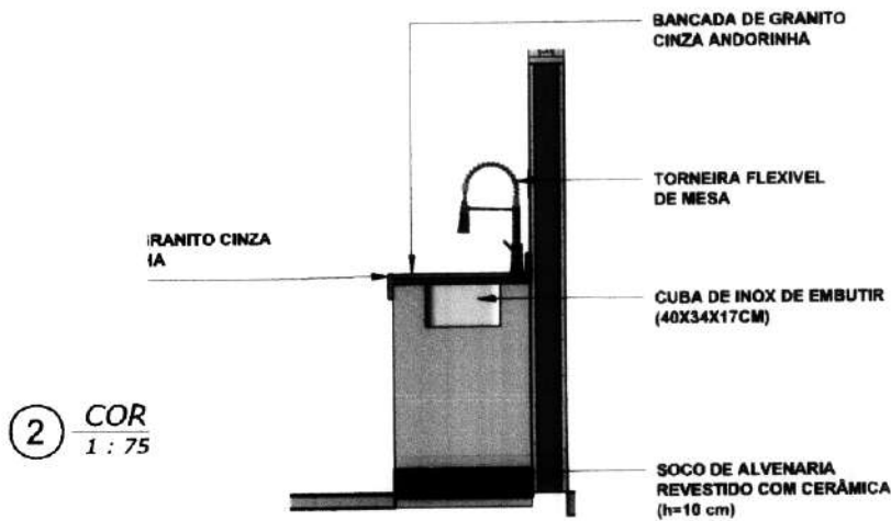
TALHE - CORTE BANCADA DE GRANITO 25
